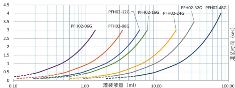
毫升泵头PFH02灌装能力曲线表
